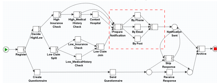
d. Model, M_4
