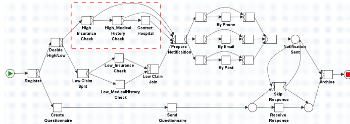
b. Model, M_2
