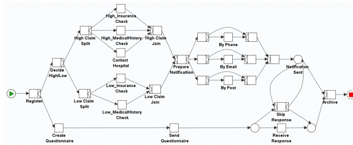
a. Model, M_1
