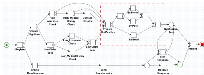
e. Model, M_5
